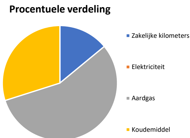
Figuur 3.2: Verdeling CO2-emissies 2016 (exclusief diesel)
